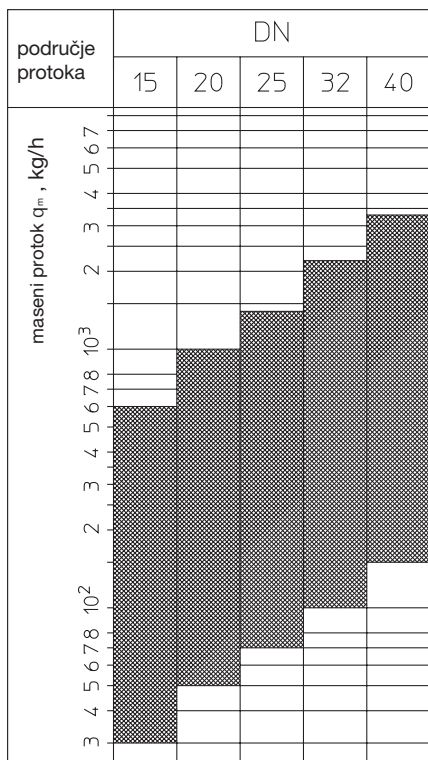
Područja protoka regulatora diferencijalnog pritiska Hyocon DP za granske diferencijalne pritiske s mogućnošću regulisanja (50 - 300, odnosno 250 - 600 mbar).
