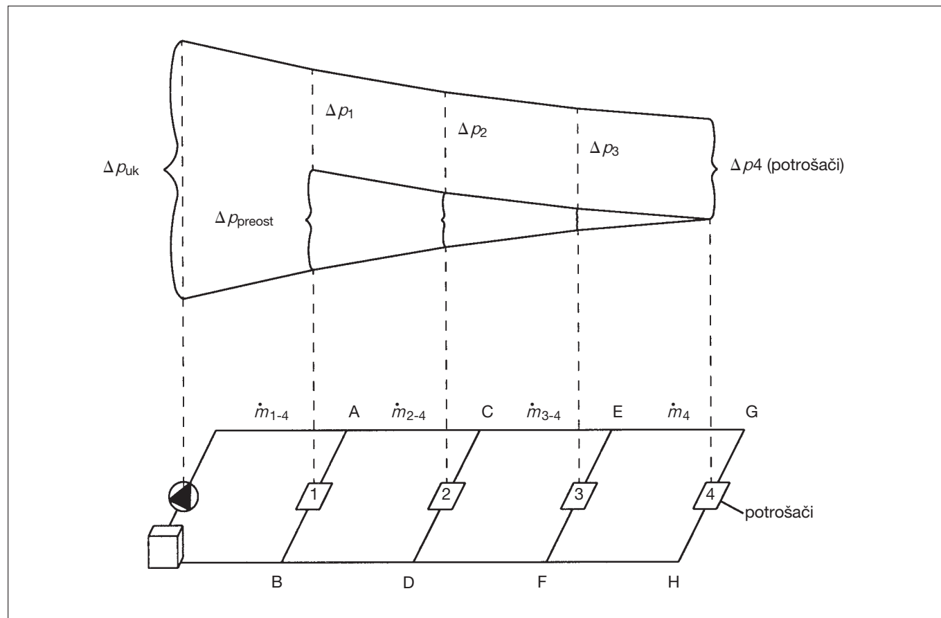
Raspodela pritiska u grani
