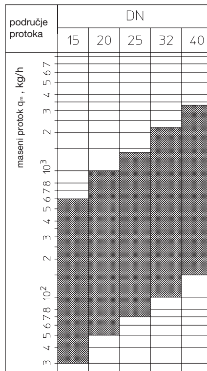
Područja protoka regulatora diferencijalnog pritiska Hyocon DP za granske diferencijalne pritiske s mogućnošću regulisanja (50 - 300, odnosno 250 - 600 mbar) i dodatno ograničenje protoka na granskom regulacionom ventilu Hyocon V.
