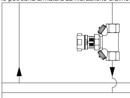
Primer: dvocevni sistem grejanja za male, odnosno srednje protoke.
