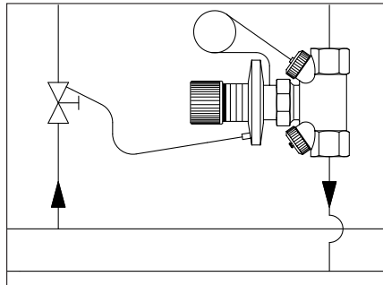
Primer: regulacija diferencijalnog pritiska u sistemima s termostatskim ventilima s mogućnošću pred-regulisanja (grane s malim, odnosno srednjim protocima).
