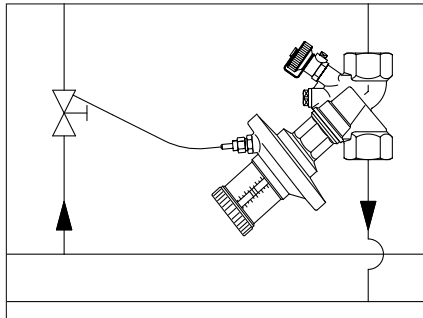
Primer: regulacija diferencijalnog pritiska u sistemima s termostatskim ventilima s mogućnošću pred-regulisanja (grane sa srednjim, odnosno velikim protocima).
