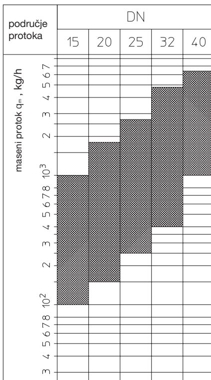
Područja protoka regulatora diferencijalnog pritiska Hydromat DP za granske diferencijalne pritiske s mogućnošću regulisanja (50 - 300 mbar).
